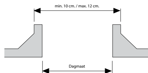
figuur 1 | Afbeelding opstand
